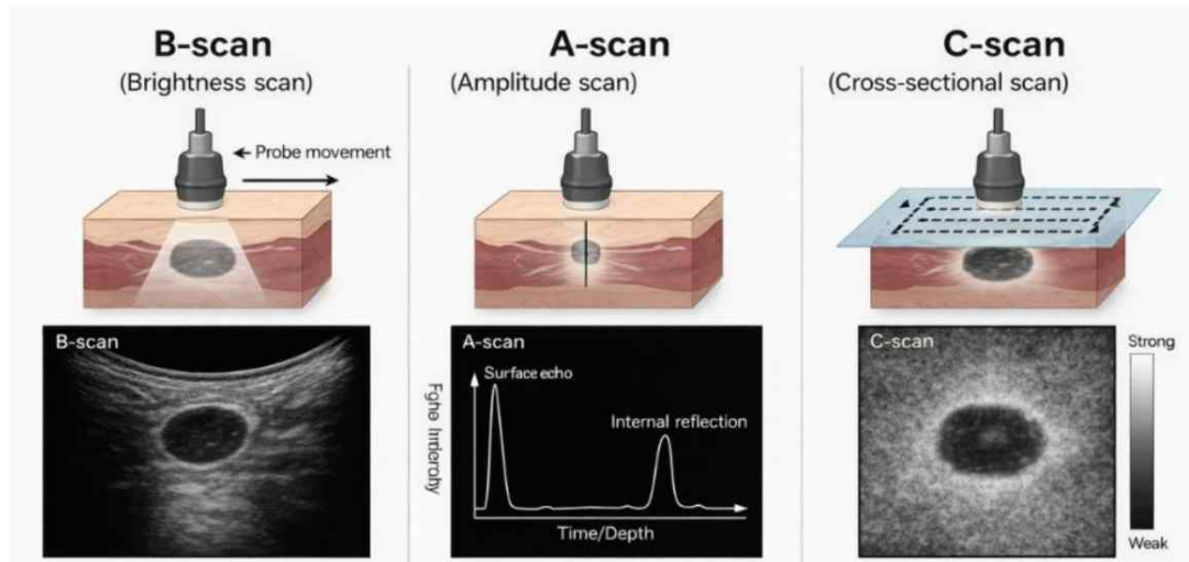
그림 3. 초음파 B-Scan / A-Scan / C-Scan 비교
