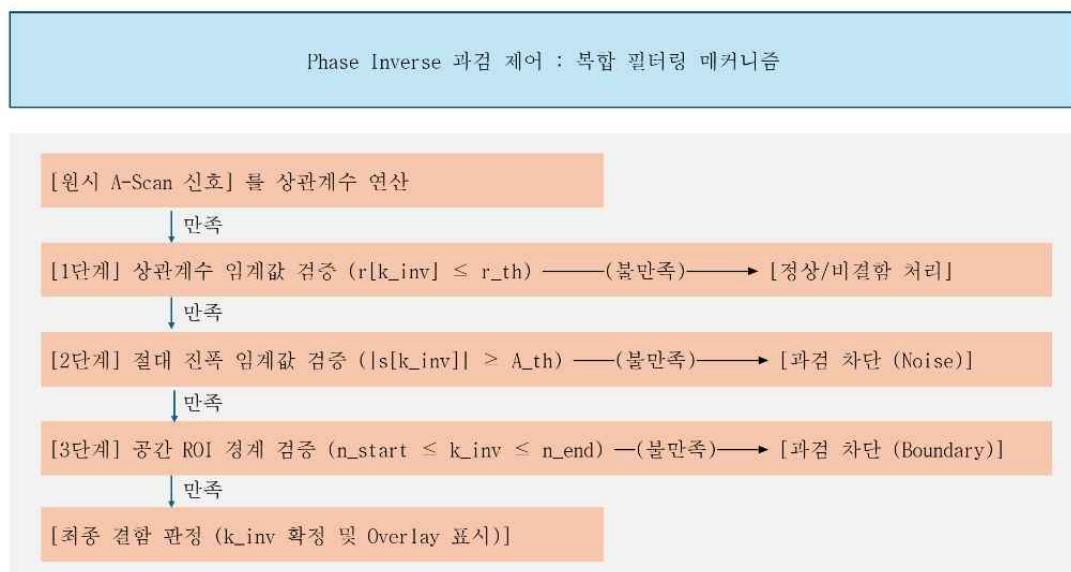
그림 6 Phase Inverse 과검 필터 연산
