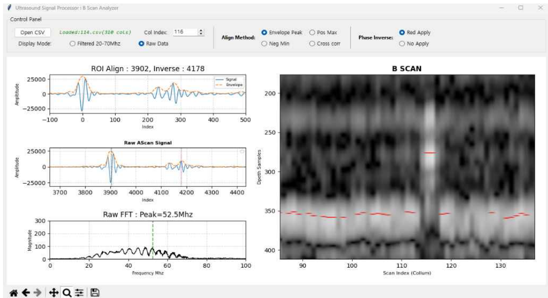
그림15. Phase Inverse 를 입힌 B-SCAN 확대 UI
