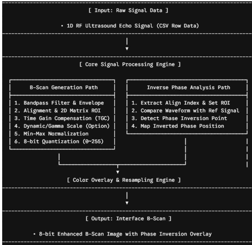
그림 10 프로그램 알고리즘
