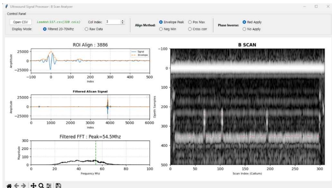
그림 12. B-Scan 및 Phase Inversion 융합 그래픽 사용자 인터페이스(GUI)
