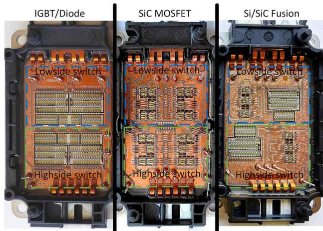
그림 1. 최신 전력반도체 모듈 내부 구조 (IGBT, SiC MOSFET, Si/SiC Fusion)
