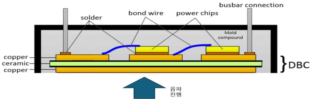
그림16. 전력반도체 내부 구조
