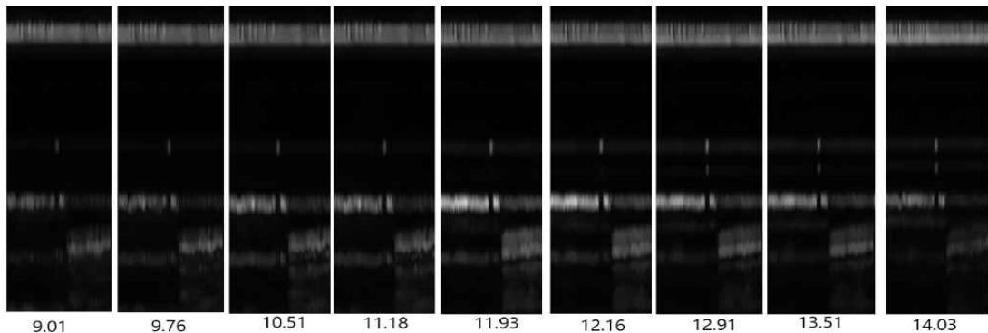
그림 13. WD 에 따른 B스캔 비교
