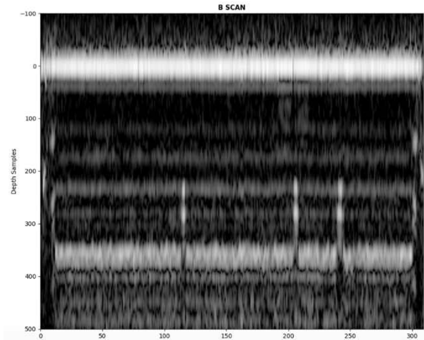
그림 7 B-스캔 영상
