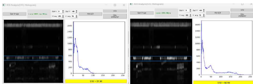
그림14. WD 9.01mm, WD 11.93mm 히스토그램 및 STD 비교
